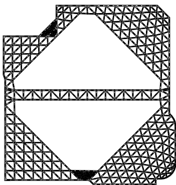
混凝土支撑平面布置图
