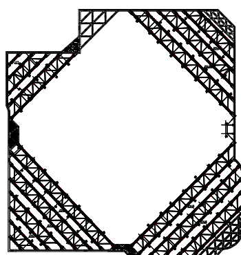
张弦梁钢支撑平面布置图
