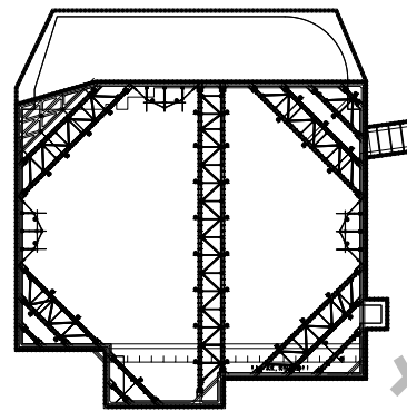
张弦梁钢支撑平面
